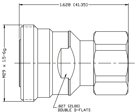
Dimensions : Inches (Millimetres)
