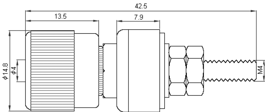
Dimensions : Millimetres
