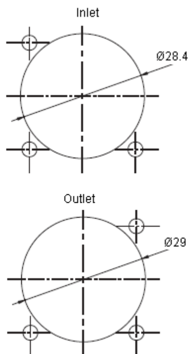
Dimensions : Millimetres
